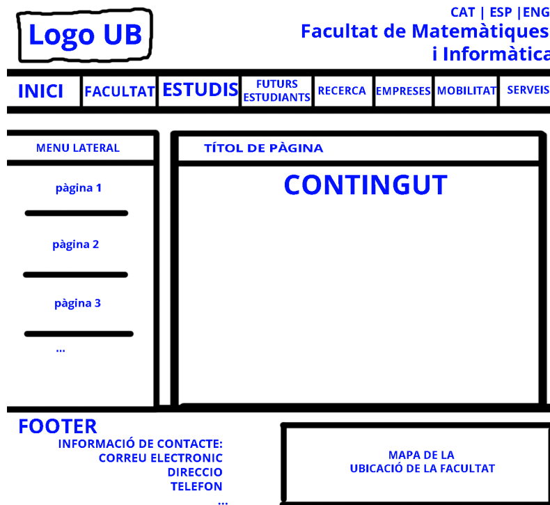
Figura 4: Disseny de plantilla d'una Pàgina Predeterminada
